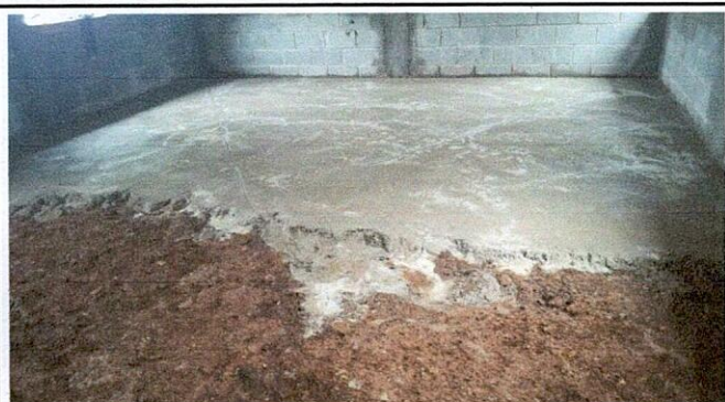
Foto: 3 MEJORAMIENTO MODULO DE AULA TIPO PORTICO, FUNDICION DE PISO
