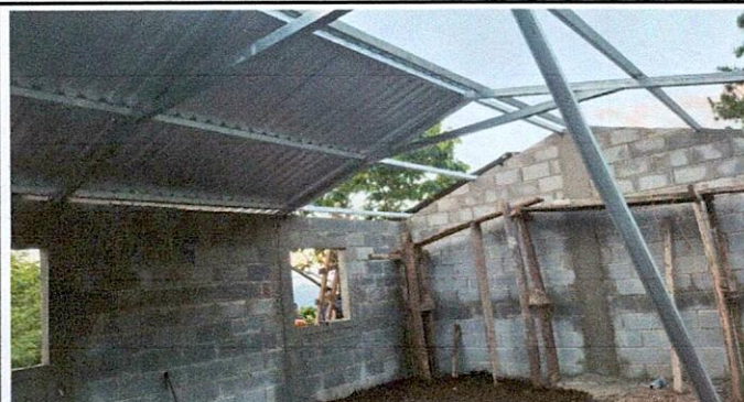
Foto: 4 MEJORAMIENTO MODULO DE AULA TIPO PORTICO, COLOCACIÓN DE LÁMINA TROQUELADA
